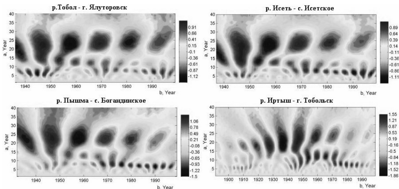
Рис. 2. Вейвлет-спектры среднегодовых расходов воды рек района «А»
