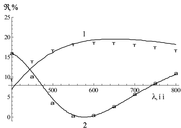
Рис. 2. Спектр отражения пленки с тремя слоями наночастиц. Точками показаны результаты численного решения, сплошной линией – расчет в рамках предлагаемого метода.
