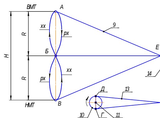
Рис. 2. Положения крайнего рычага 9 четырёхзвенного шарнирно-рычажного механизма Уатта
