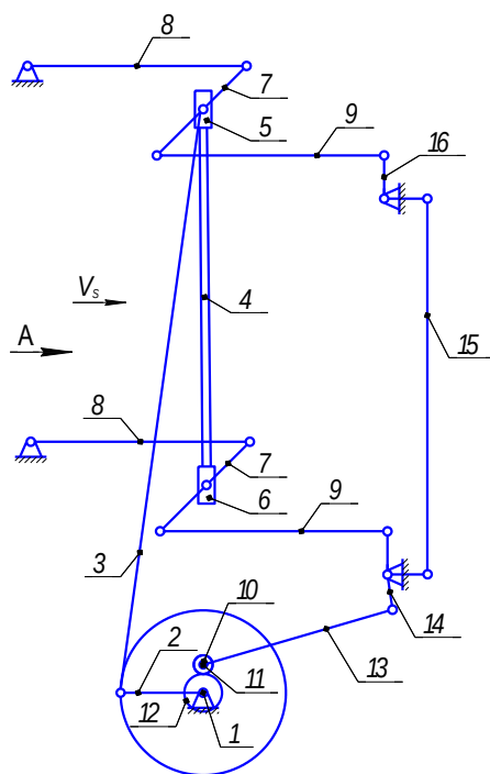
Рис. 1. Принципиальная схема лесопильной рамы с рычажной подвеской и качанием пильной рамки по самопересекающейся замкнутой кривой типа восьмерки
