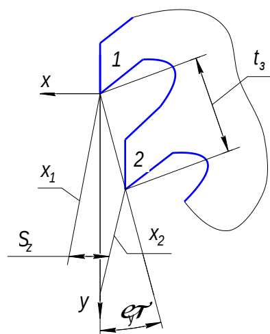
Рис. 3. Схема перемещения зубьев пилы в пропиле
