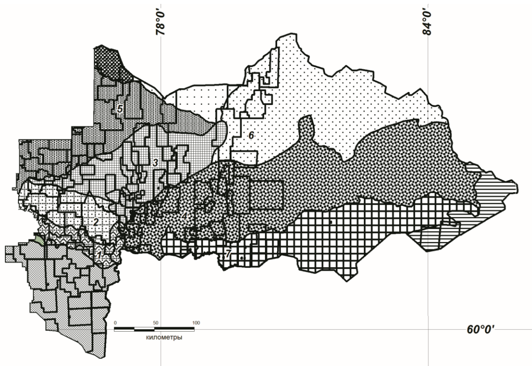
Рис. 1. Карта – схема ключевых участков
