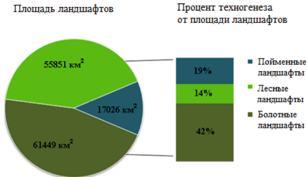
Рис. 2. Соотношение площади естественных и техногенных ландшафтов
