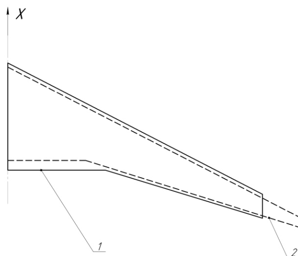
Рис. 8. Геометрическая интерпретация изменения величины эффективного удлинения для крыла с ДАП: 1 – крыло магистрального ВС с ДАП; 2 – эквивалентное крыло без ДАП
