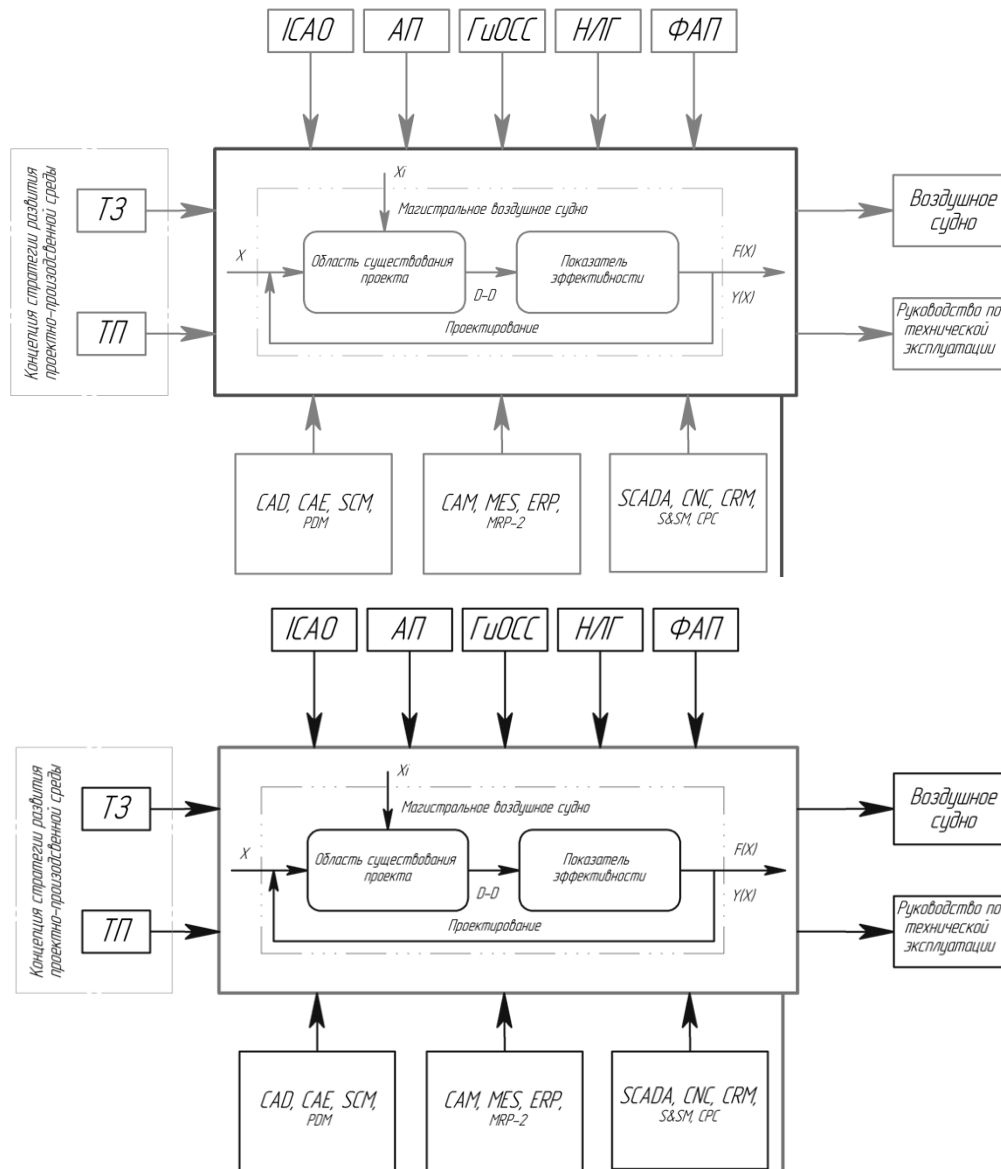
Рис. 3. Внешнее проектирование магистрального ВС
