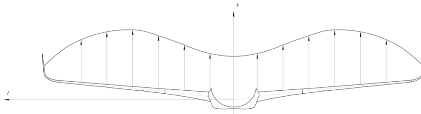
Рис. 10. Распределения подъемной силы вдоль размаха крыла магистрального ВС с ДАП, тип «Крылышко»
