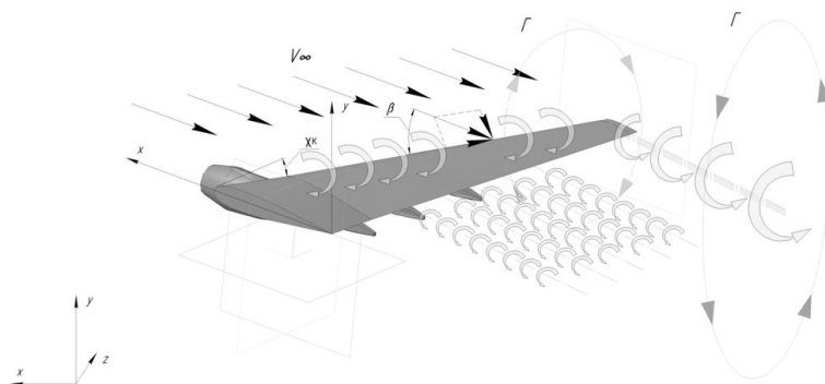
Рис. 12. Картина обтекания крыла бесконечным потоком со скоростью V_\infty магистрального ВС без ДАП
