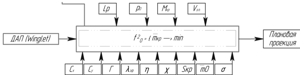
Рис. 5. Проектирование элементов магистрального ВС, «Крыло + ДАП»
