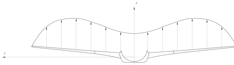
Рис. 9. Распределения подъемной силы вдоль размаха крыла магистрального ВС без ДАП
