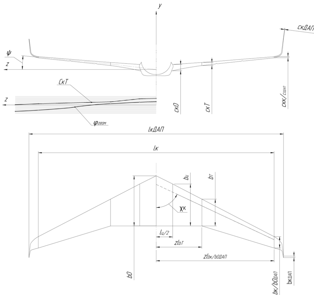
Рис. 6. Параметризованная плановая проекция крыла с ДАП магистрального ВС тип «Крылышко»
