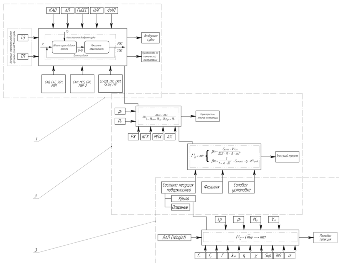
Рис. 7. Логико-структурная схема синтеза проектных решений с детализацией проектных процедур для крыла магистрального ВС: 1 – внешнее проектирование (предварительное, предпроектные исследования); 2 – эскизное проектирование; 3 – проектирование элементов ВС
