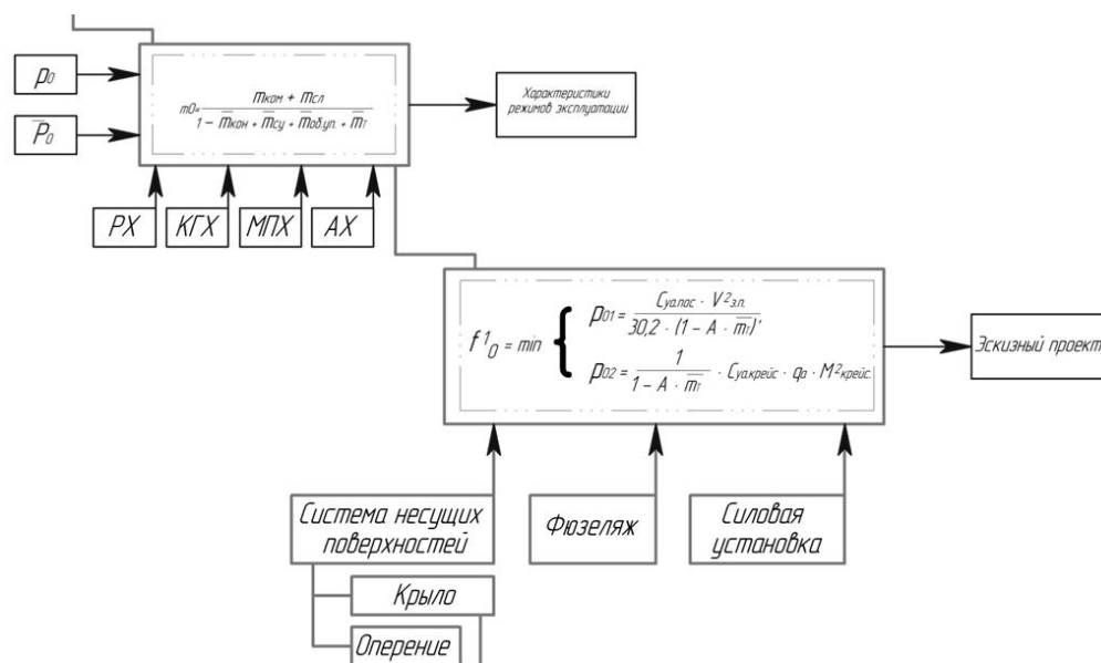
Рис. 4. Эскизное проектирование магистрального ВС
