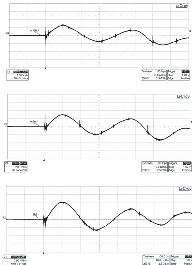
Рис. 4. Кривые разрядного тока «I» при энергиях разряда батареи конденсаторов W: 0,3; 0,5; 1 кДж. Значения W, I и H приведены в таблице 3
