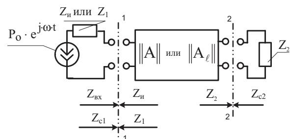
Рис. 2. Расчётная схема трубопроводной системы. Импедансы источника колебаний и нагрузки «приведены» к сечениям «1-1» и «2-2»
