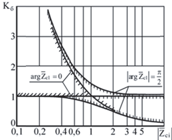
Рис. 5. Зависимости предельных значений коэффициента K_6 при различных значениях аргумента волнового сопротивления гасителя
