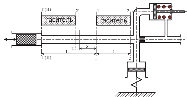
Рис. 1. Схема трубопроводной системы и варианты размещения гасителя
