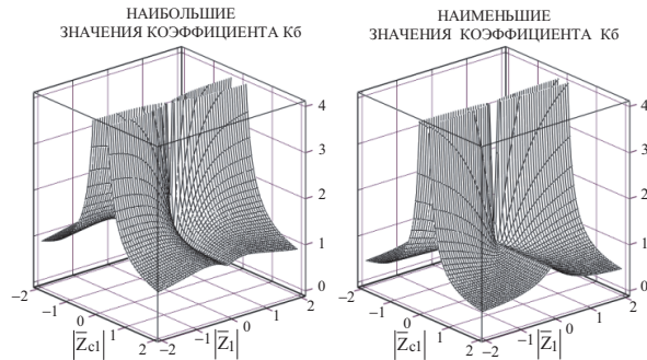
Рис. 4. Зависимости наибольших и наименьших значений коэффициента K_6 от изменений импеданса источника колебаний и волнового сопротивления гасителя, обращённого в сторону источника колебаний
