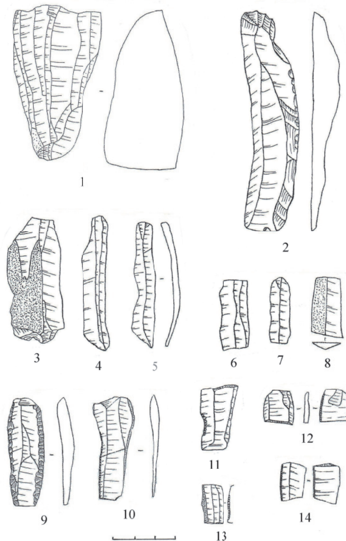
Рис. 2. Евстюниха I. Изделия из камня (1 – нуклеус; 2 – комбинированное орудие; 3–8 – пластины без ретуши; 9–14 – пластины с вторичной обработкой)
