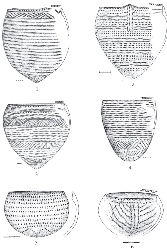
Рис. 1. Евстюниха I. Реконструкция неолитических сосудов (1–6; по: Герасименко А.А., 2008)
