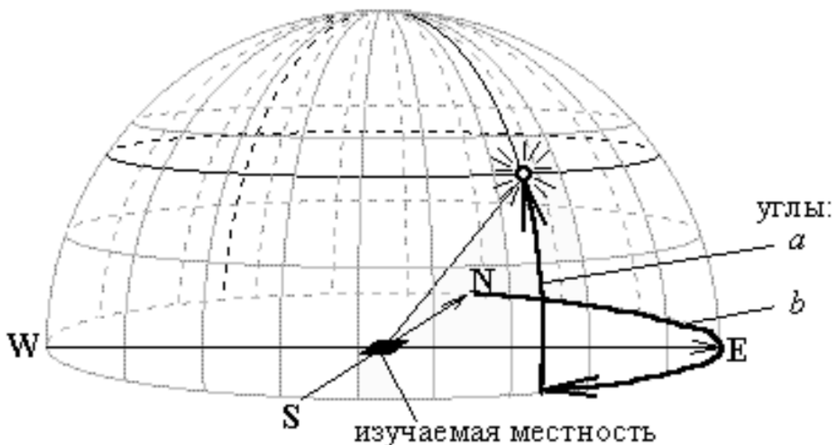
Рис.4. Два угла, a и b , определяющих положение Солнца на небосводе. a есть склонение Солнца от горизонта, b есть азимут Солнца.
