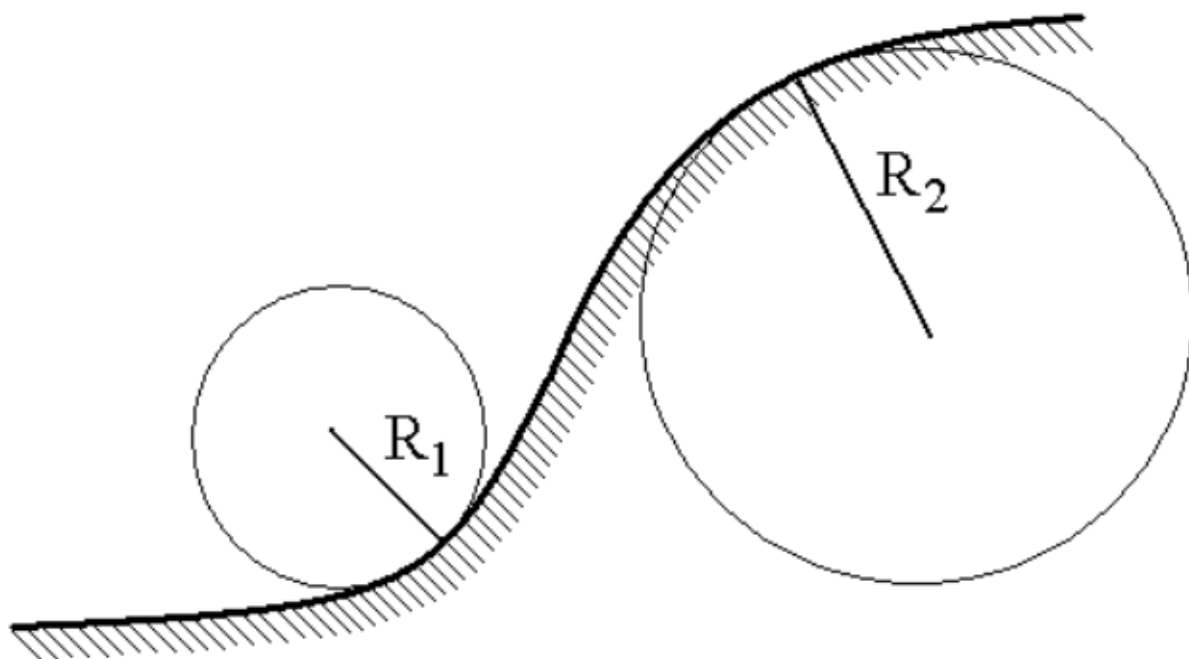
Рис.2. Схема профиля склона для пояснения вертикальной кривизны k_v . Радиусы кривизны R имеют разные знаки для выпуклого ( R_2 > 0 ) и вогнутого ( R_1 < 0 ) участков профиля склона, а k_v = 1/R .
