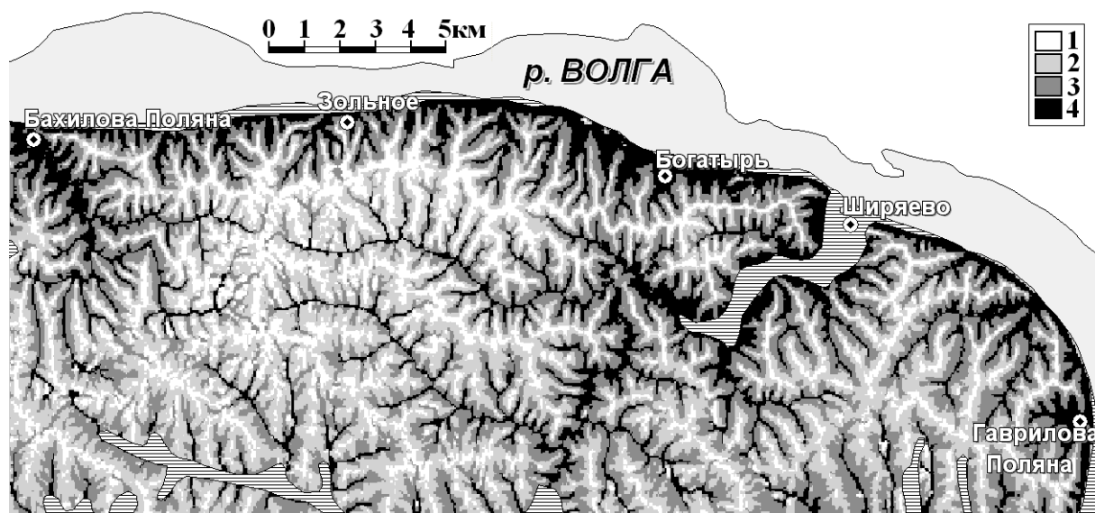
Рис. 8. Изображение карты-матрицы типов местоположения экосистемы Жигули: 1-элювиальный, 2-трансэлювиальный, 3-транзитный, 4-транаккумулятивный и аккумулятивный типы.
