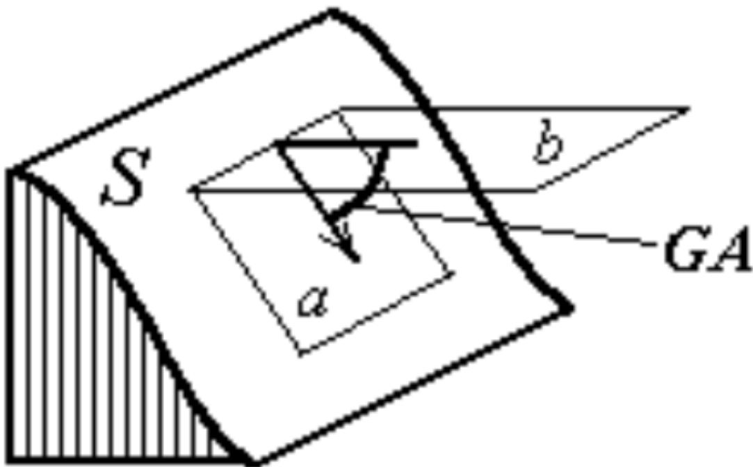
Рис.1. Крутизна склона рассчитывается как угол уклона GA между горизонтальной и касательной поверхностями.
