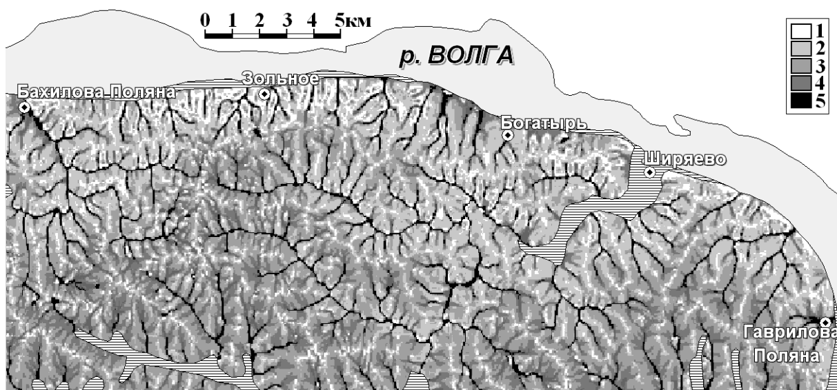
Рис. 9. Изображение карты-матрицы гранулометрического состава почвообразующих пород:
