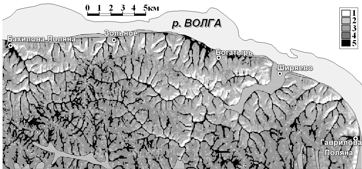
Рис. 10. Изображение карты-матрицы типов местообитания экосистемы Жигули:
