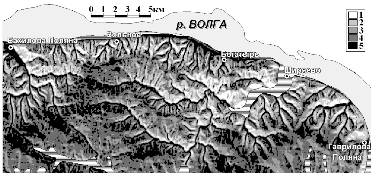
Рис. 11. Изображение карты-матрицы мощности гумусового профиля. Мощность в см: 1 – 5-16; 2 – 16-32; 3 – 32-40; 4 – 40-45; 5 – 45-97.
