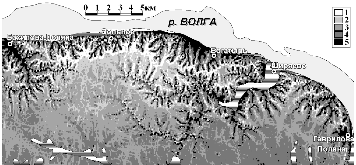
Рис. 12. Изображение карты-матрицы индекса упругой устойчивости. Индекс в долях единицы: 1 – 0,05-0,25; 2 – 0,25-0,35; 3 – 0,35-0,45; 4 – 0,45-0,65; 5 – 0,65-0,95.
