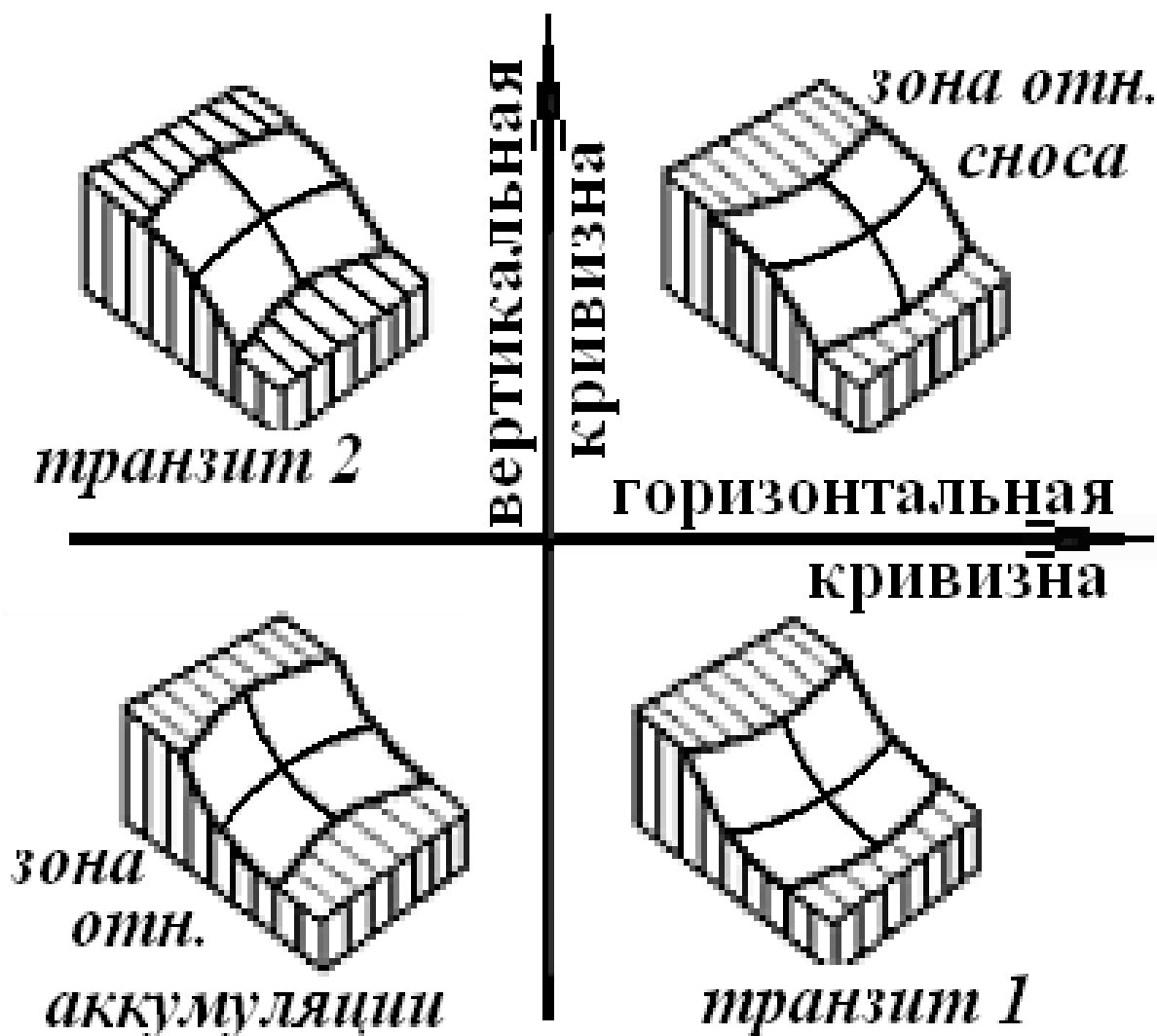
Рис.3. Классификация форм рельефа по знакам горизонтальной и вертикальной кривизн (Troeh, 1964).
