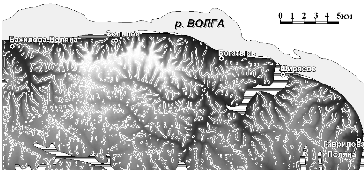
Рис. 7. Приводораздельные области Самарской Луки, площадь сбора менее 0,25 га (показаны белыми контурами).
