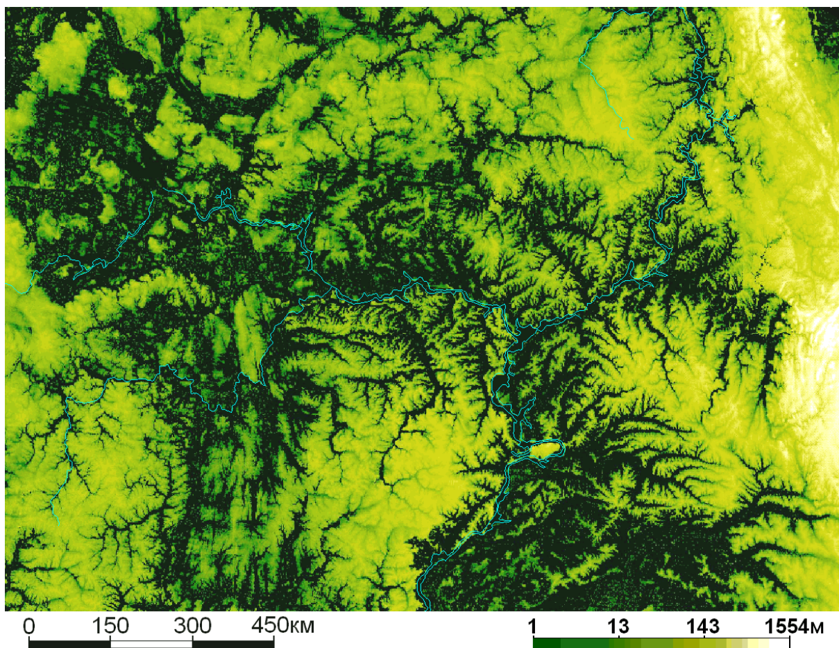
Рис. 5. Общий вид В-холмов Среднего Поволжья (рис.5а):
