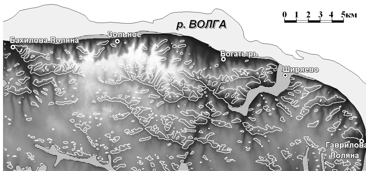
Рис. 6. Области сильной освещенности (показаны белыми контурами).
